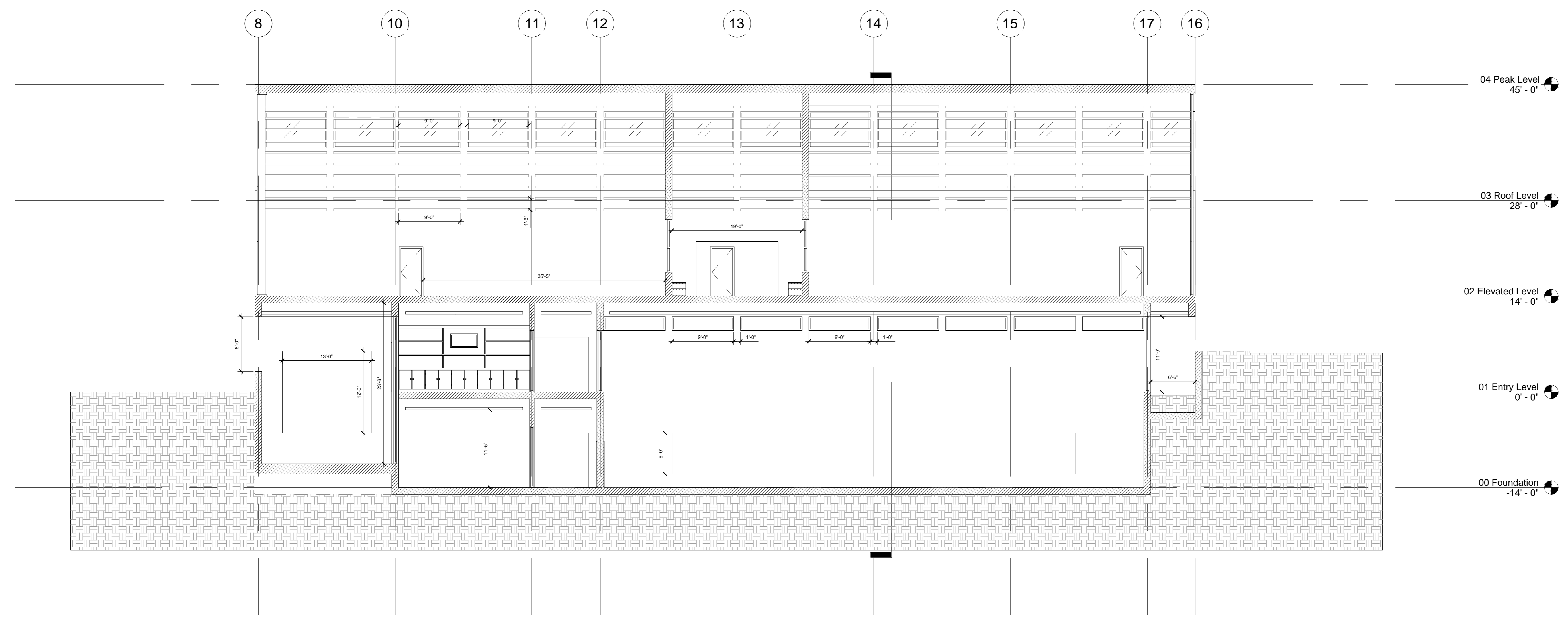
1 Longitudinal Section A251 Scale 1/8" = 1'-0"
